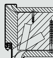
Obvodová zárubňa montáž do muríva hmoždinové kotvy do muríva
