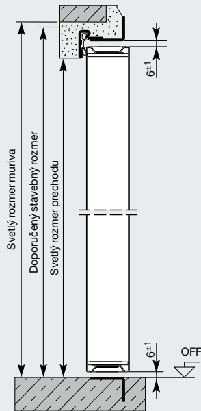
Zobrazenie bez dorazového uholníka
