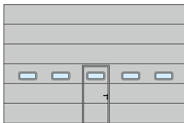
SPU F42 Lamelové okná typ A umiestnenie integrovaných dverí v strede
