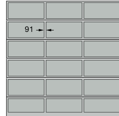
ALR F42 Vitraplan rovnomerné rozdelenie polí
