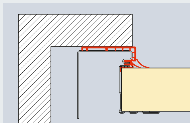
Bočný doraz s ThermoFrame
