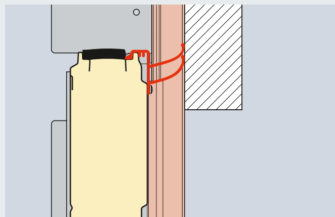
Prekladový doraz s ThermoFrame
